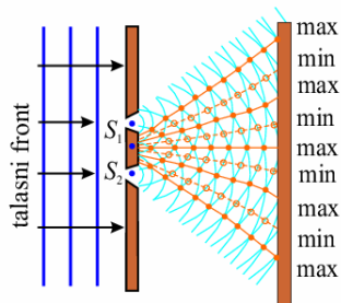
Slika 12.28: Širenje svetlosti iz dva proreza i njena interferencija.
