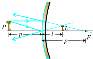
Slika 12.20: Konstrukcija lika kod rasipnih ogledala.
