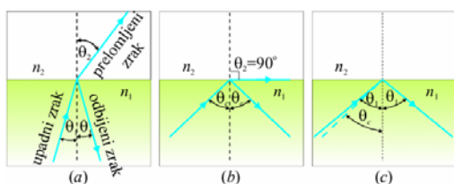
Slika 12.5: Uz objašnjenje efekta totalne refleksije.
