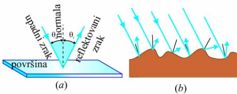
Slika 12.1: Ilustracija zakona odbijanja (a) koji важи за сваки (ravni) delić neravne površine (b).
