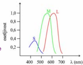
Slika 12.23: Relativna osjetljivost tri tipa čepića na različite talasne dužine.
