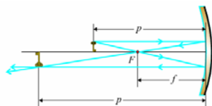
Slika 12.18: Konstrukcija lika kod sabirnog ogledala za p > f .
