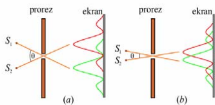
Slika 12.35: Difrakcione slike dva različito udaljena tačkasta izvora. Ugao \theta se naziva ugaona odvojenost predmeta.
