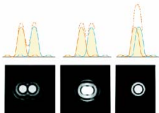
Slika 12.36: Difrakcione slike dva različito udaljena tačkasta izvora.
