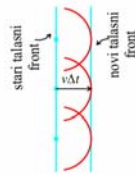
Slika 12.24: Хајгенсов принцип.
