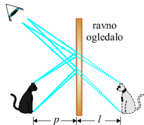
Slika 12.15: Konstrukcija lika kod ravnog ogledala.
