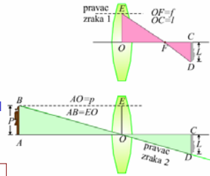
Slika 12.12: Sabirno sočivo.
