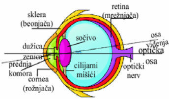
Slika 12.22: Šematski prikaz preseka oka.
