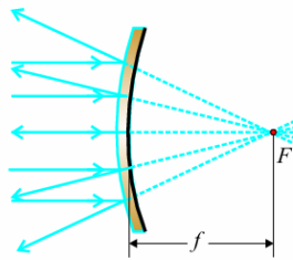
Slika 12.17: Konveksno sferno ogledalo.
