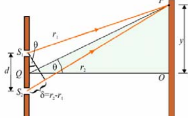
Slika 12.30: Razlika pređenih puteva talasa iz dva proreza koji dolaze u istu tačku na zaklonu.
