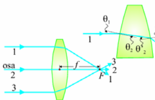
Slika 12.9: Sabirno sočivo.
