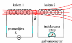
Slika 11.24: Promene u prvom kalemu indukuju elektromotornu silu u drugom.
