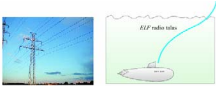
Slika 11.31: (a) Dalekovi. (b) Da bi talas mogao da dodje do podmornice mora da ima veoma veliku talasnu dužinu, odnosno ekstremno nisku frekvenciju (ELF).
